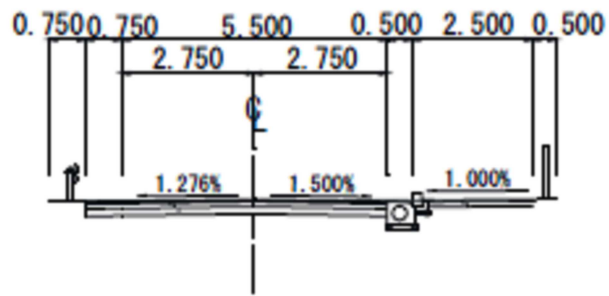
標準断面図
