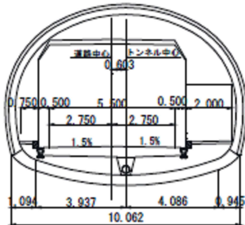
トンネル部
