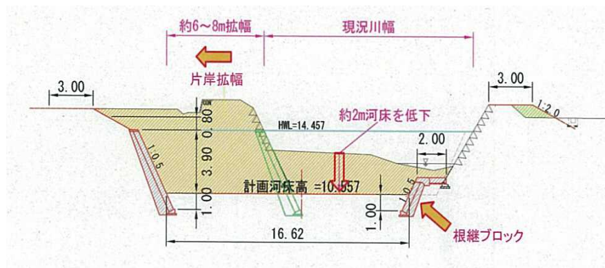
断面図
